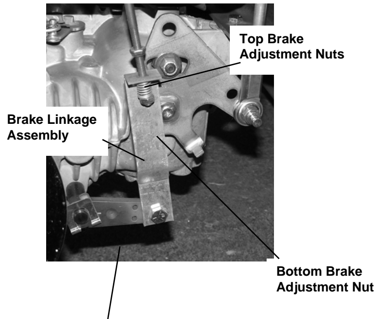
Brake Rod Arm
